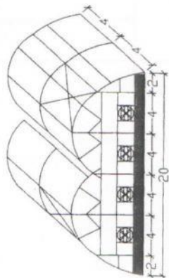
Fan Side Elevation
